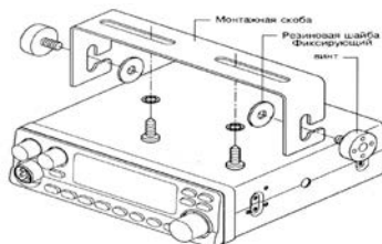
Рис.1. Крепление радиостанции при помощи монтажной скобы.
